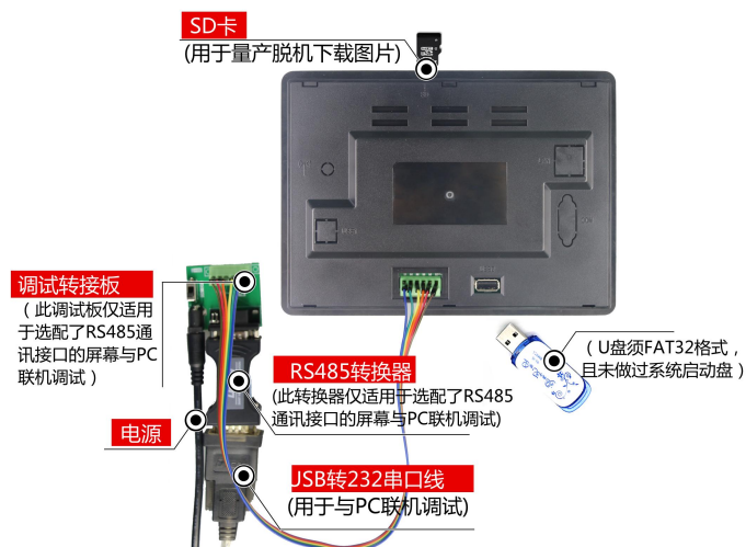
图 1-3 RS485 调试图
