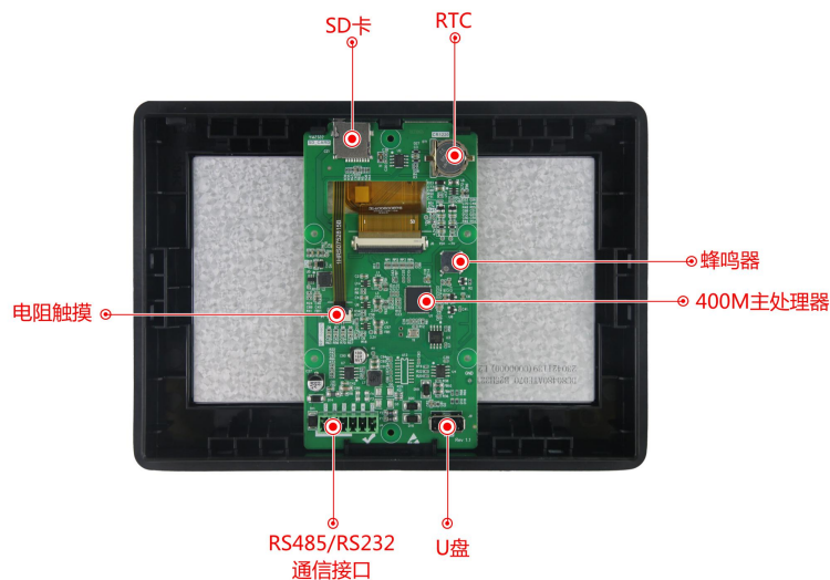
图 1-2 硬件配置图
