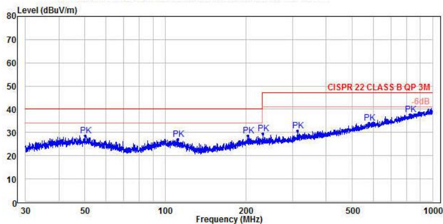
图 7-6 辐射测试水平方向
