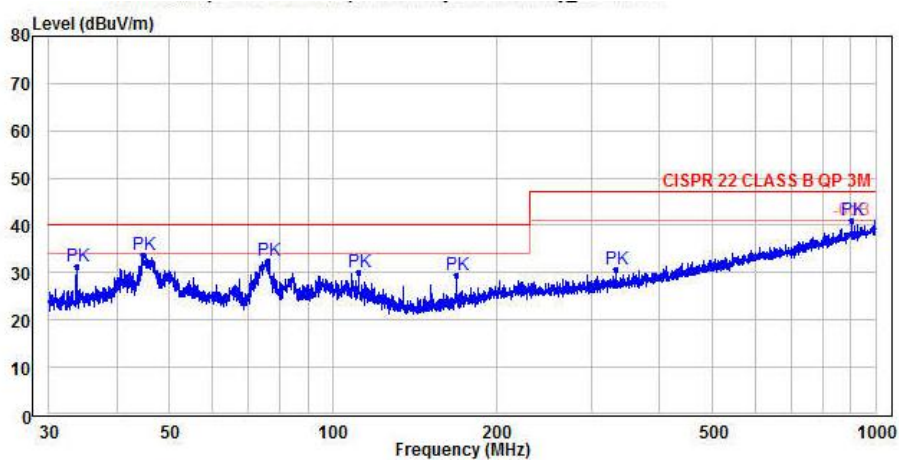
图 7-7 辐射测试垂直方向
