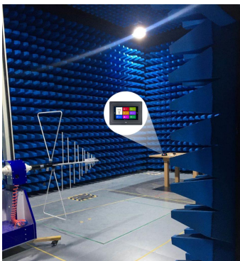
图 7-5 辐射测试图
