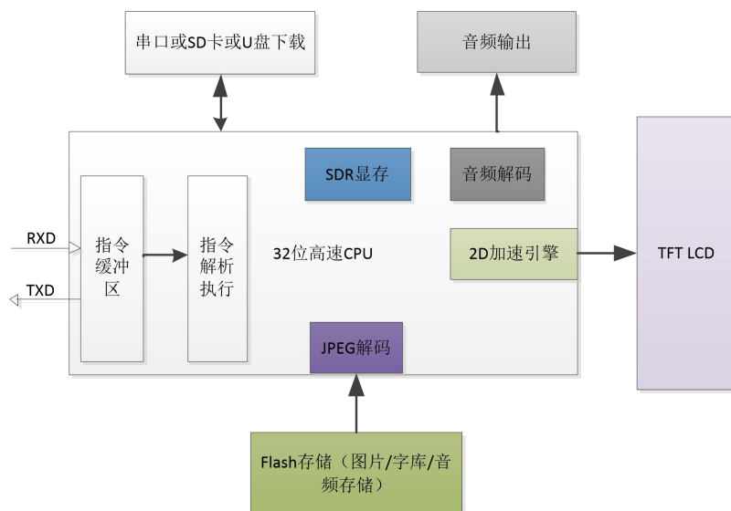
图 11-1 HMI 硬件结构参考图
